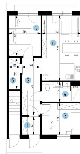
Rzut mieszkania
